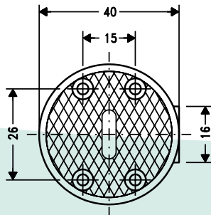
Zeichnung: Rechtsschloß Drawing: right door Plan: porte à droite
